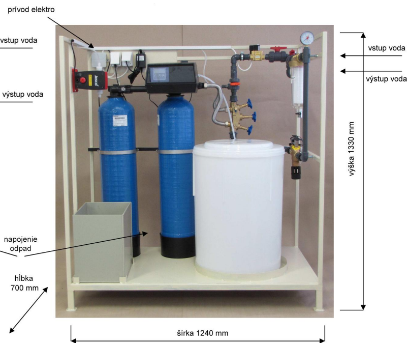
BUV s duplexným ( príp. jednoduchým ) zmäkčovacím filtrom
